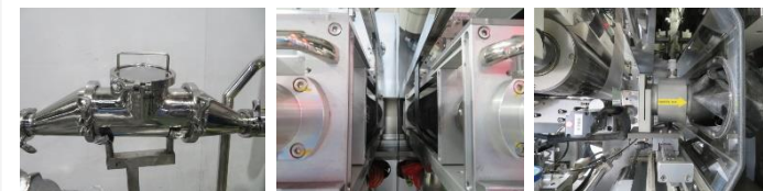
磁性过滤器
